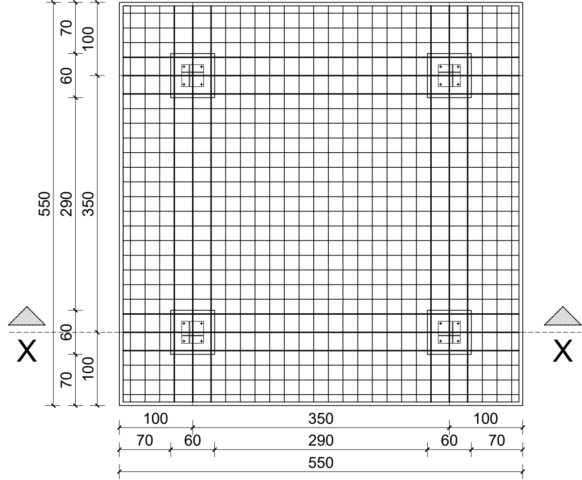
PIANTA ARMATURA PLINTO - scala 1:50
