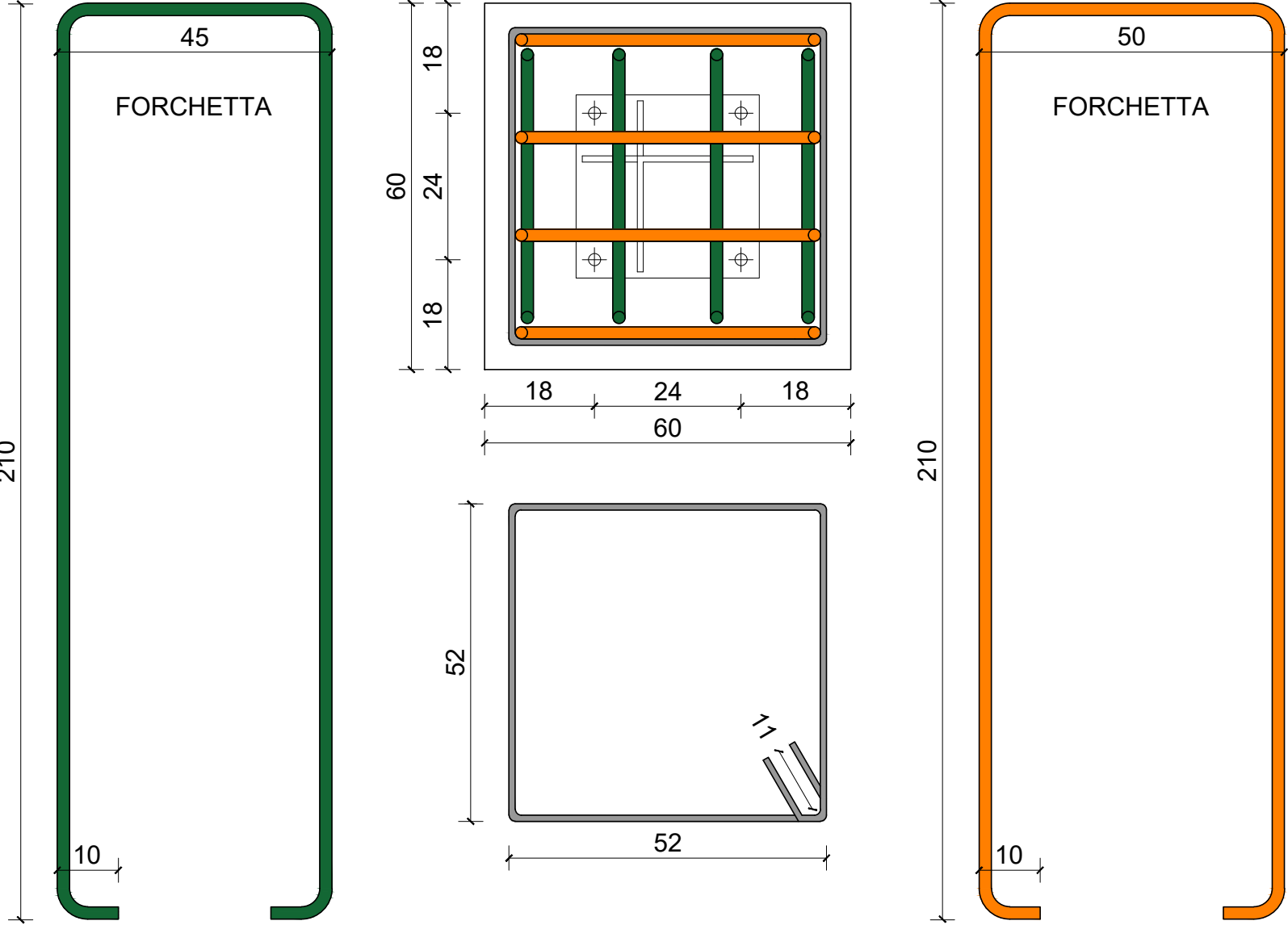
PIANTA ARMATURA APPOGGIO - scala 1:10
