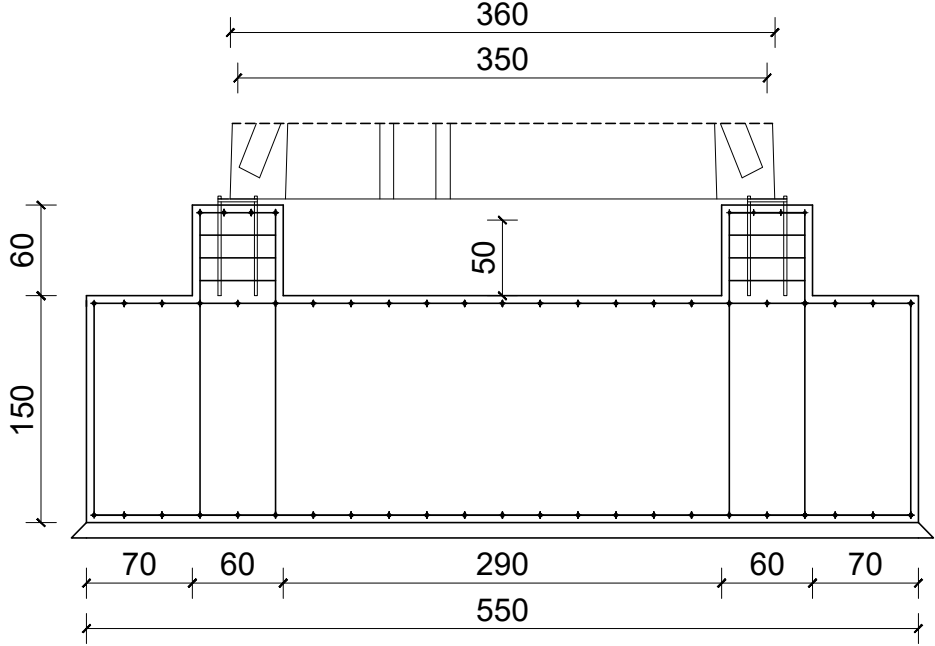
PIANTA ARMATURA APPOGGIO - scala 1:10
