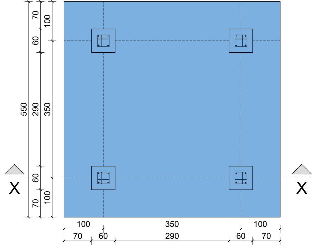
PIANTA PLINTO - scala 1:50
